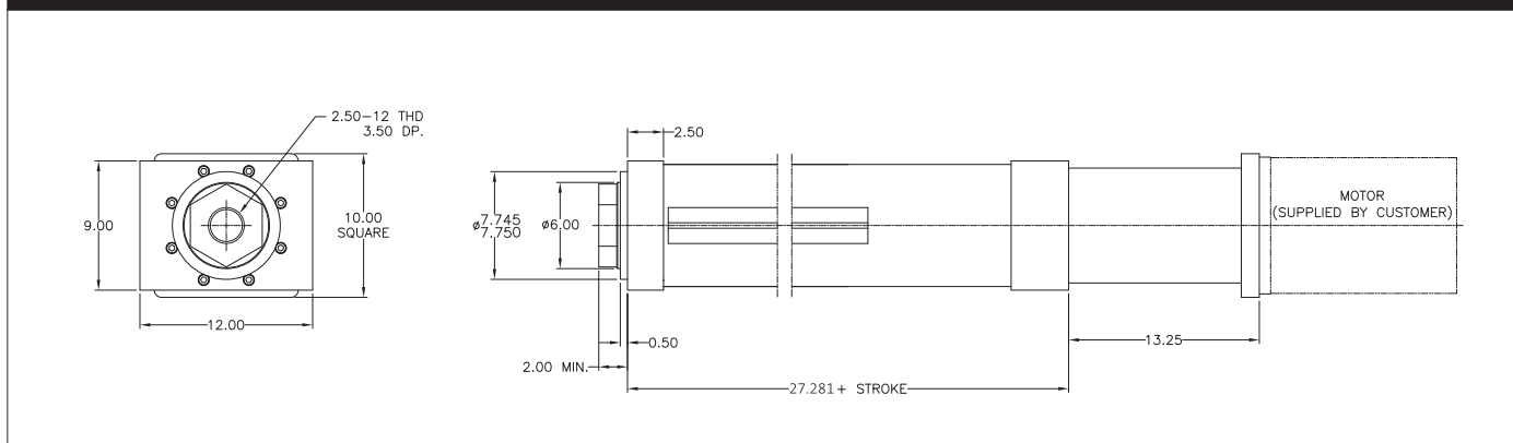
L-Inline Motor Dimensions
