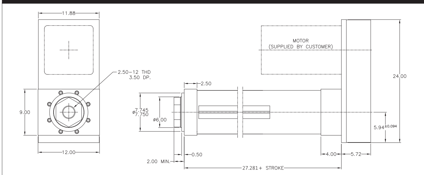
L-Inline Motor Dimensions
